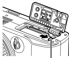
Кнопка защелки аккумулятора
