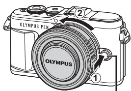
Objektiventriegelung
