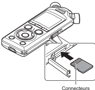
Connecteurs
