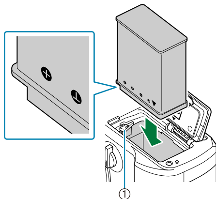
① 电池锁扣
