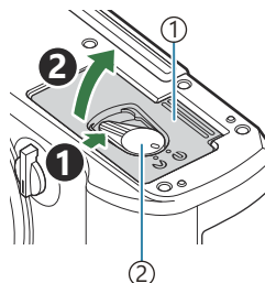
① Cobertura do compartimento da bateria ② Bloqueio do compartimento da bateria
